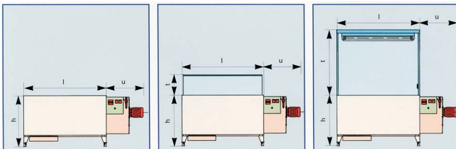
Schleiftisch mit Kabinenaufsatz für optimale Stauberfassung
